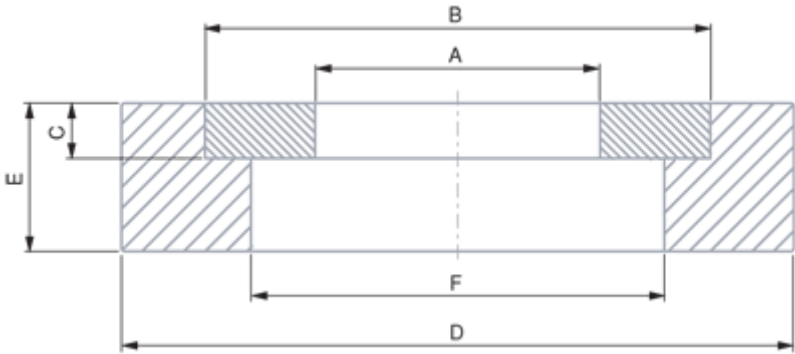
Габаритные размеры
